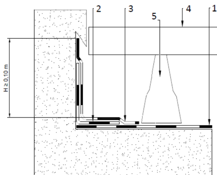
Figure 5 – Toitures-terrasses accessibles dalles sur plots Niveau fini des dalles au-dessus de la tête des relevés
