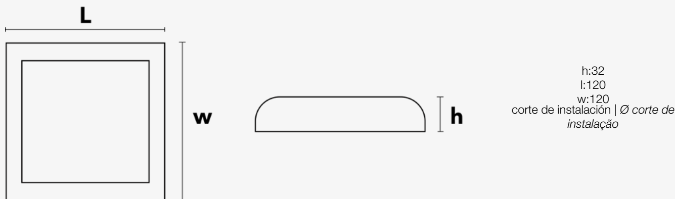
Esquema de Producto. Product line drawing
