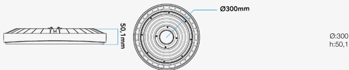
Esquema de Producto. Product line drawing
