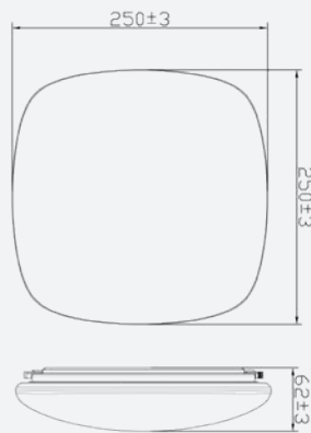
Esquema de Producto. Product line drawing
