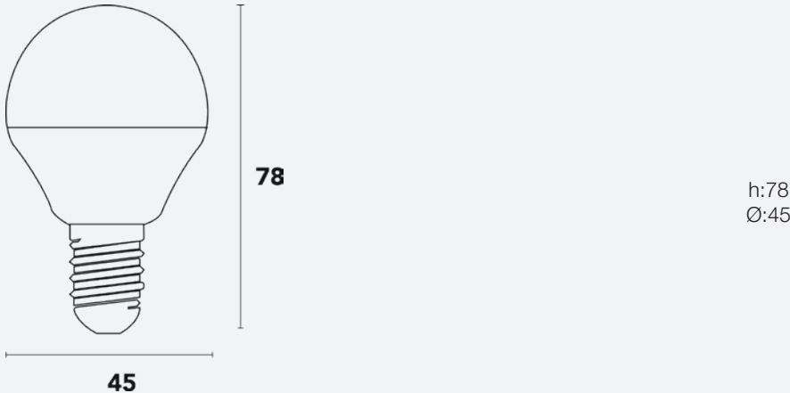
Esquema de Producto. Product line drawing
