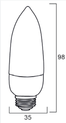
Esquema de Producto. Product line drawing
