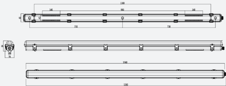
Esquema de Producto. Product line drawing
