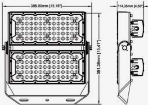
Esquema de Producto. Product line drawing
