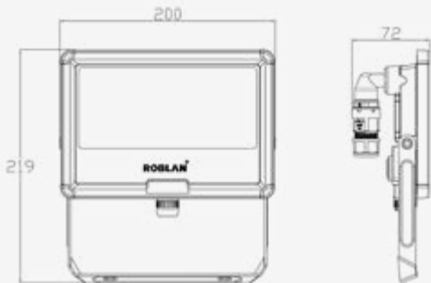
Esquema de Producto. Product line drawing
