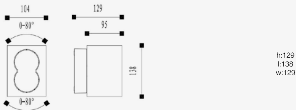
Esquema de Producto. Product line drawing
