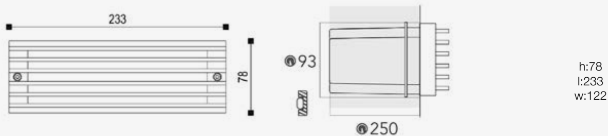
Esquema de Producto. Product line drawing
