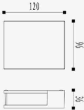
Esquema de Producto. Product line drawing
