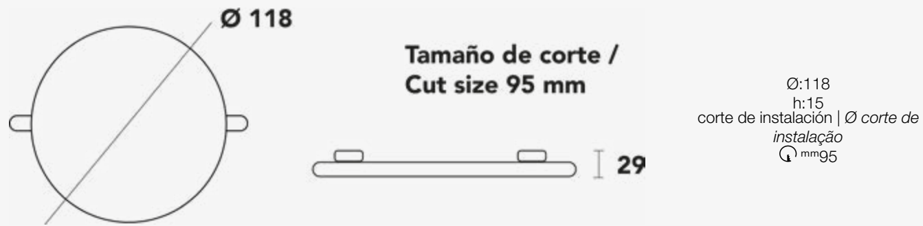
Esquema de Producto. Product line drawing
