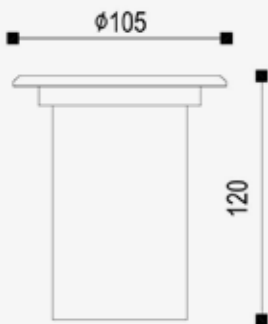
Esquema de Producto. Product line drawing
