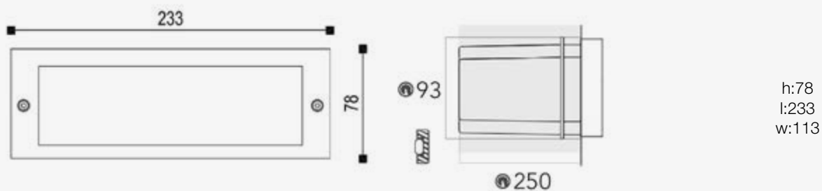
Esquema de Producto. Product line drawing
