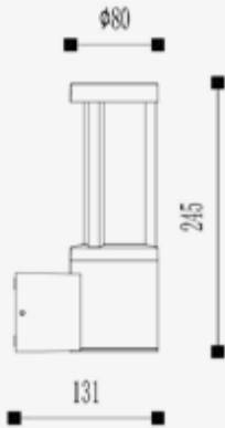
Esquema de Producto. Product line drawing
