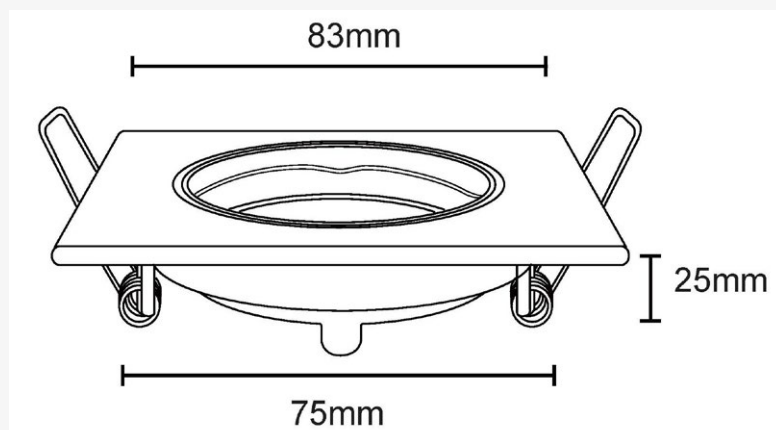
Esquema de Producto. Product line drawing
