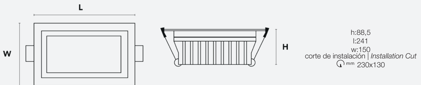
Esquema de Producto. Product line drawing
