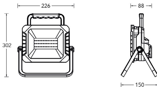
Esquema de Producto. Product line drawing
