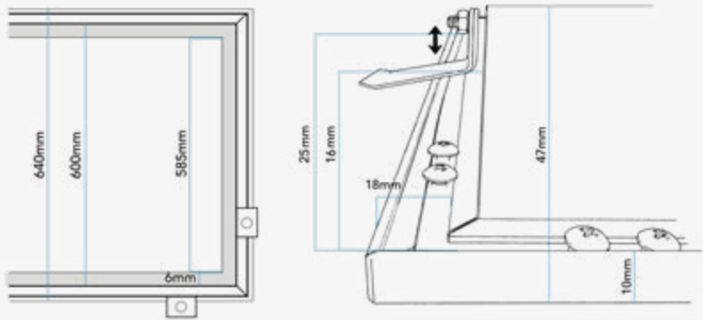
Esquema de Producto. Product line drawing
