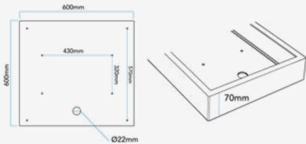
Esquema de Producto. Product line drawing
