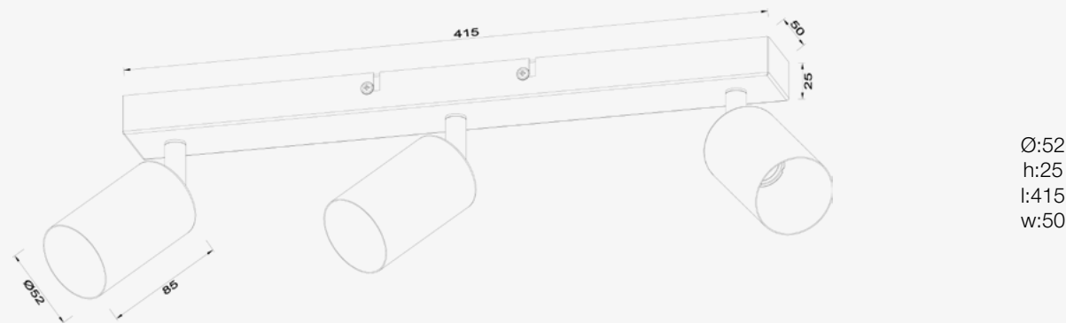
Esquema de Producto. Product line drawing
