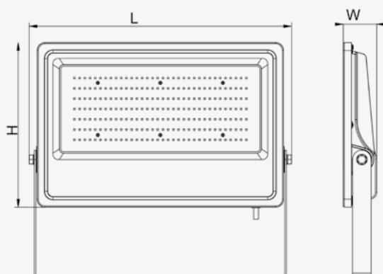
Esquema de Producto. Product line drawing
