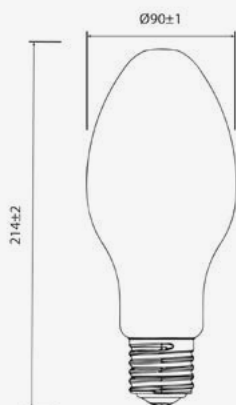
Esquema de Producto. Product line drawing
