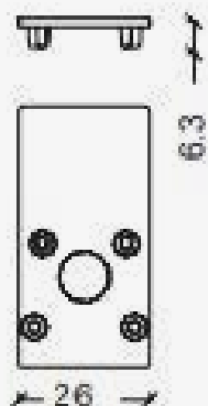
Esquema de Producto. Product line drawing
