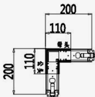
Esquema de Producto. Product line drawing
