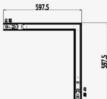
Esquema de Producto. Product line drawing
