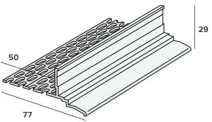
Ventilatie startprofiel nr. 2826
