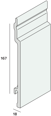
Sponningdeel fijne nerf nr. 4065
