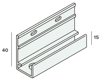
Omrandingprofiel nr. 2809
