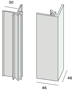
Basis uitwendig hoekprofiel nr. 2803
