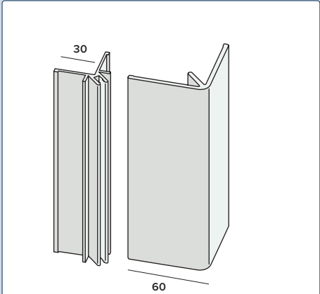
Basis uitw. hoekprofiel nr. 2803
