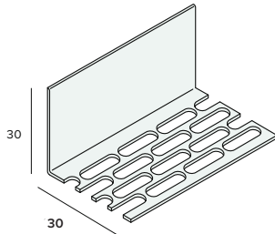
Geventileerd hoekprofiel nr. 0132
