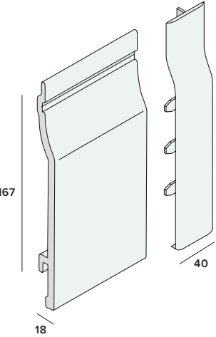
Rabat (enkel) fijne nerf nr. 4010
