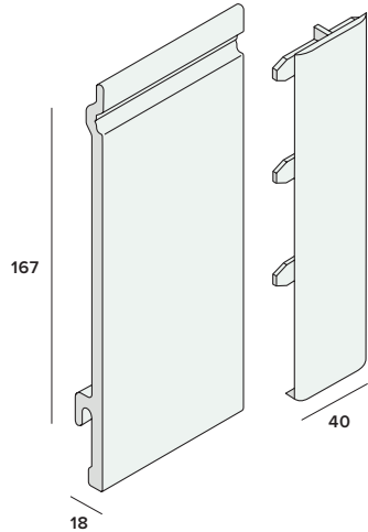
Potdeksel grove nerf nr. 4030
