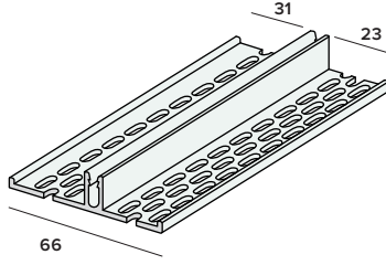
Tweezijdig ventilatieprofiel nr. 2882
