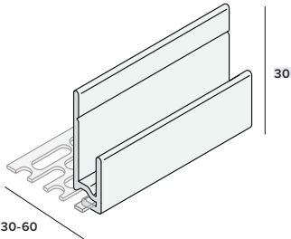
Inhaak startprofiel nr. 2808
