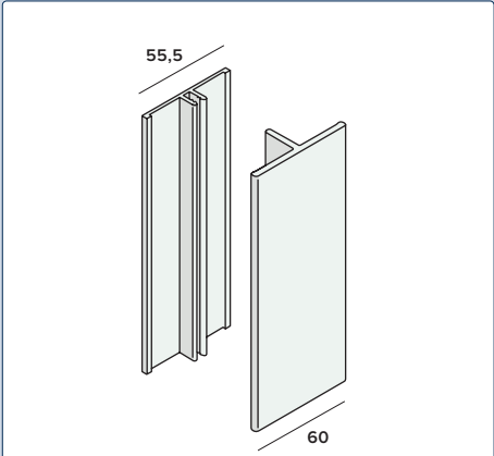
Basis verbindingprofiel nr. 2805
