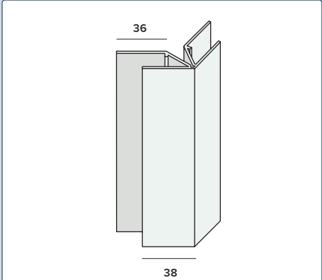
Flexibel hoekverb. profiel nr. 4089
