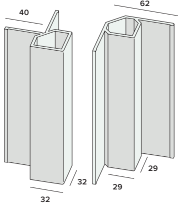
Uitwendig hoekprofiel nr. 2828
