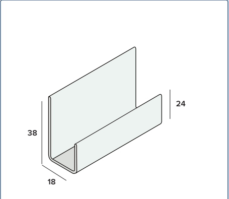
Omrandingprofiel nr. 4082
