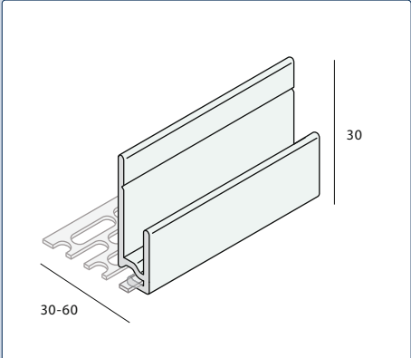
Inhaak startprofiel nr. 2808
