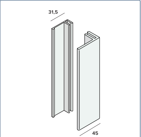
Basis eindprofiel nr. 2807
