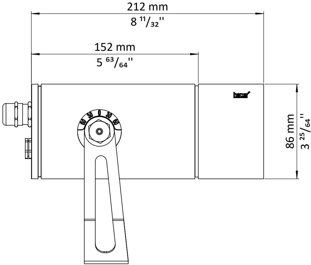
VEGA S (1-10V, DALI)
