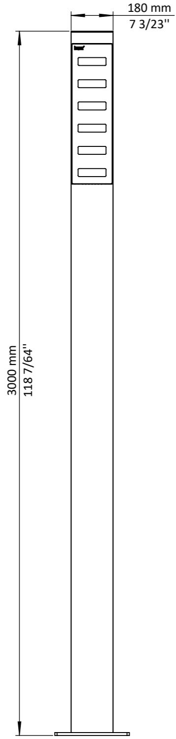
Ön Görünüş
