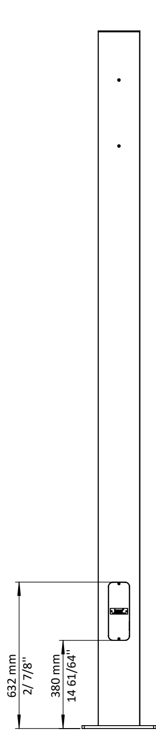
Arka Görünüş
