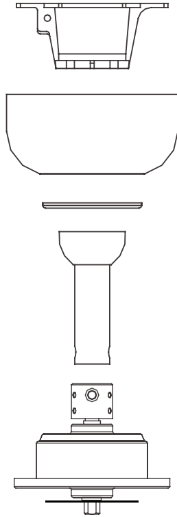
Tilt blocker for flat ceiling. Dispositif anti-basculement pour plafond plat.
