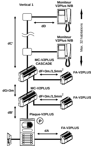
Installation avec multiplexeur en cascade et moniteurs N/B
