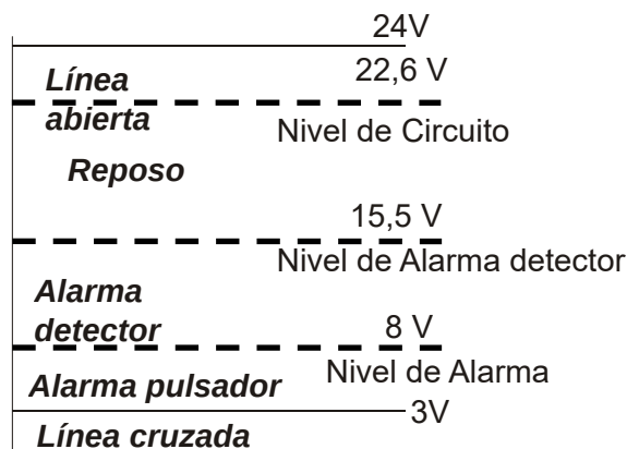
Figura 8: Umbrales de tensión de las zonas.
