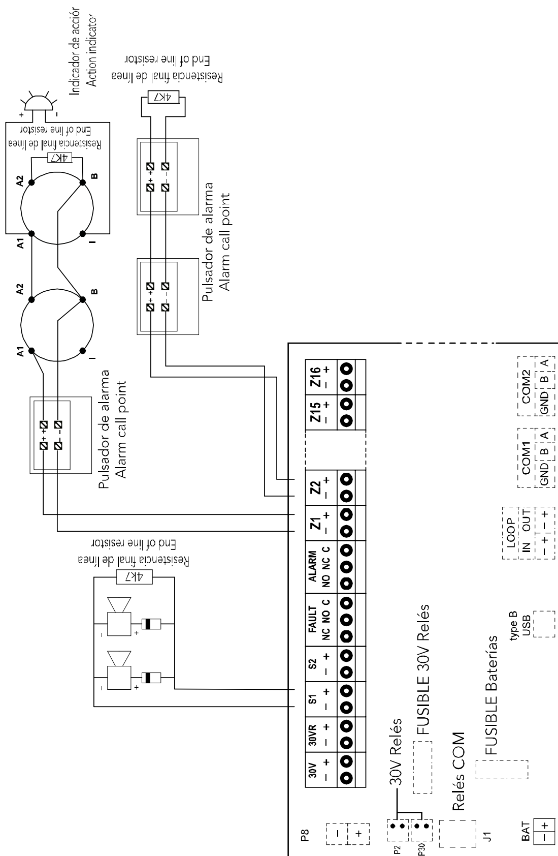
Figura 5: Esquema de conexionado de las salidas de sirena general y zonas
