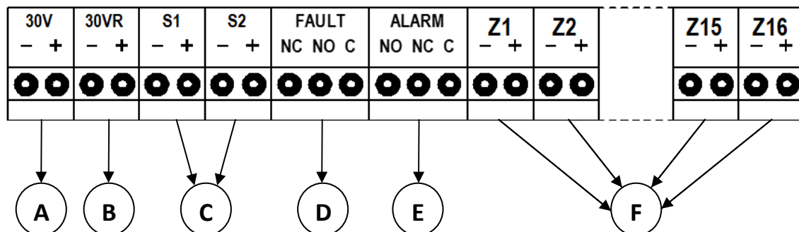
Figura 4: Esquema de los conectores de la central CCG-XXZPLUS.
