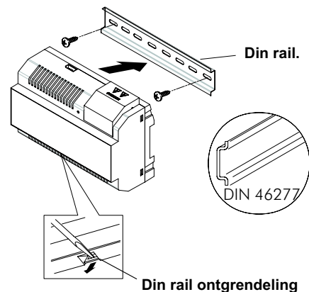
Din rail ontgrendeling
