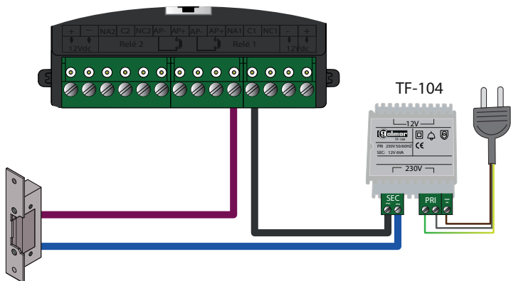
Abrepuertas máx. 12Vca/850mA
