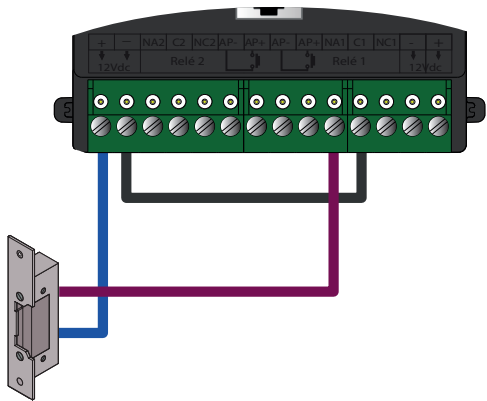
Abrepuertas máx. 12Vcc/270mA
