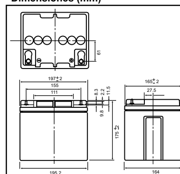
Dimensiones (mm)
