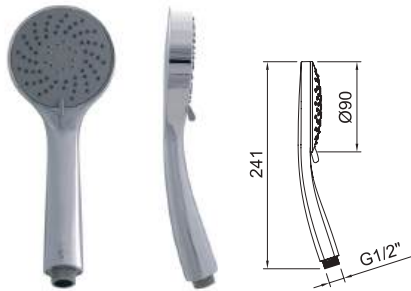
Teléfono ducha Mar Ø90mm. Mar shower handset Ø90mm.
