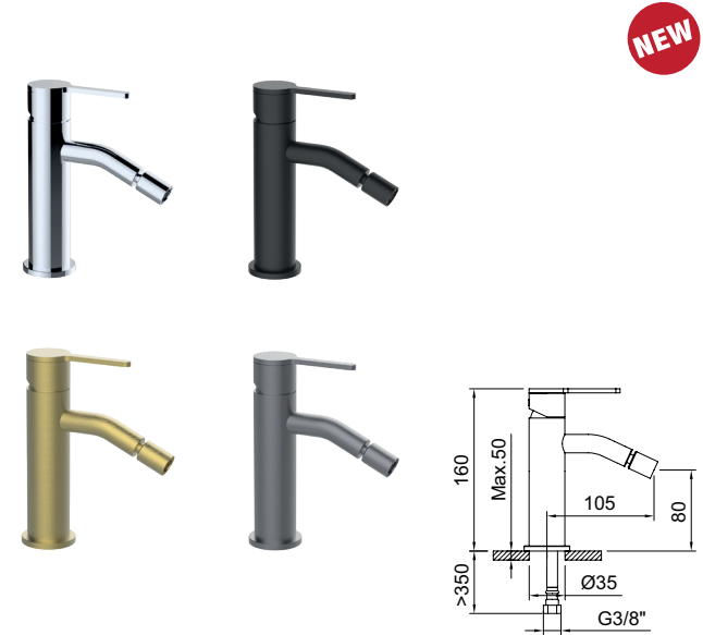
Mitigeur bidet avec aérateur rotule et flexibles de raccordement 3/8" >350mm. Single-lever bidet mixer with swivel aerator and flexible hoses 3/8" >350mm.
