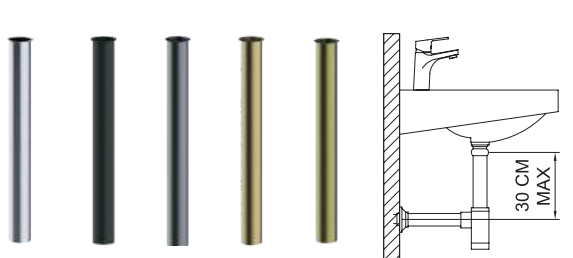
Extension pour siphon. Bottle trap extension.
