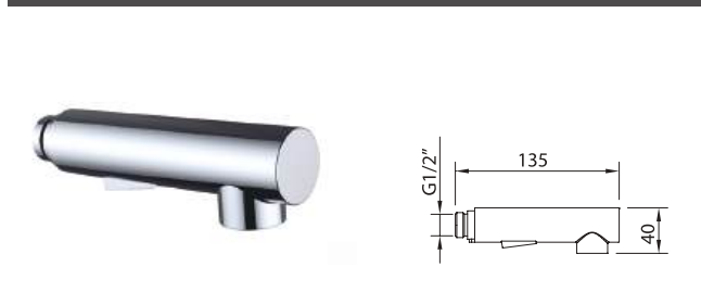
Douchette pour mitigeur évier. Pull-out handshower for sink mixer.
