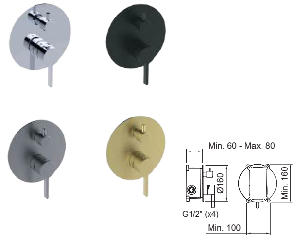
Mitigeur douche encastré 1/2". Concealed single-lever shower mixer 1/2".
