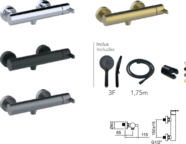
Mitigeur douche. Single-lever shower mixer.
