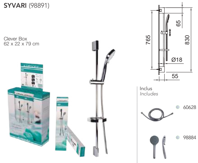
Ensemble de douche avec barre Ø18x830mm avec support articulé coulissant et porte-savon Box. Shower set with Ø18x830mm bar with sliding articulated support and soap dish holder Box.
