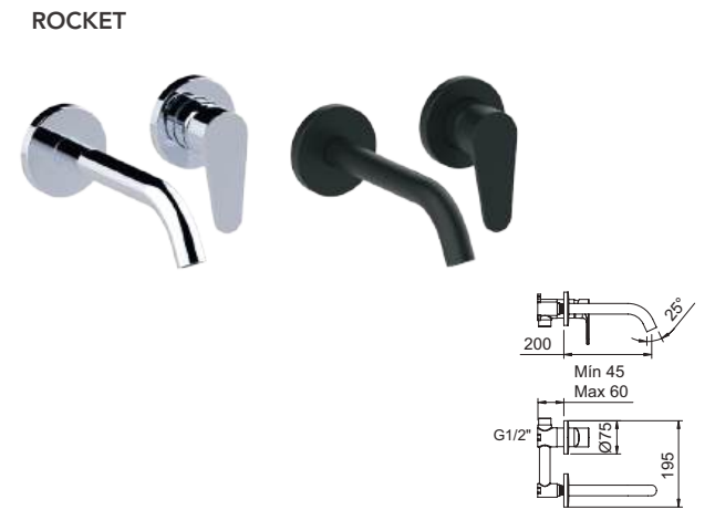
Mitigeur lavabo encastré 1/2" avec aérateur. Concealed basin mixer 1/2" with aerator.
