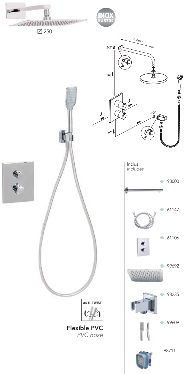
Ensemble de douche thermostatique encastré. Concealed thermostatic shower set.
