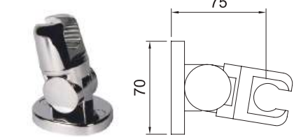
Soporte teléfono de ducha articulado. Articulated handset holder.
