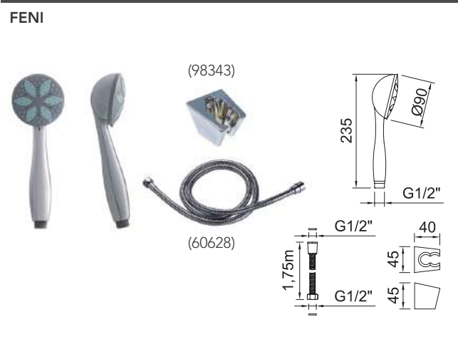
Kit de ducha Feni Ø90mm. Feni shower set Ø90mm.
