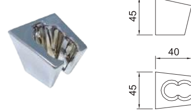
Soporte teléfono de ducha fijo. Fix handset holder.
