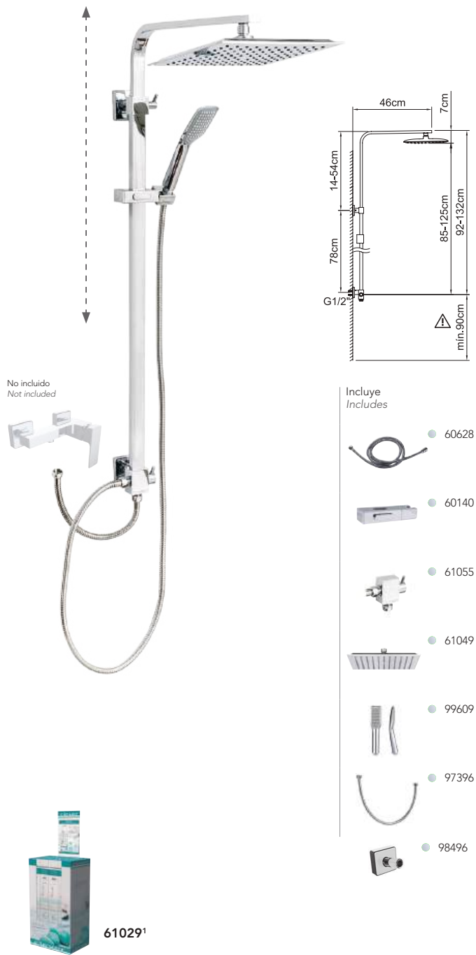
Conjunto de ducha con barra extensible con soporte articulado deslizante. Shower set with extendable bar with sliding articulated support.
