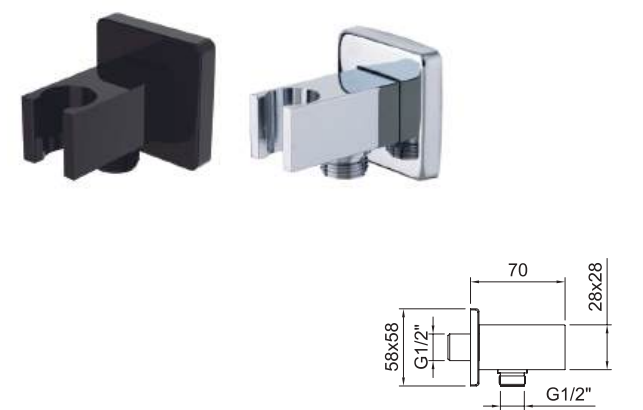
Salida flexo mural con soporte. Wall hose outlet with holder.
