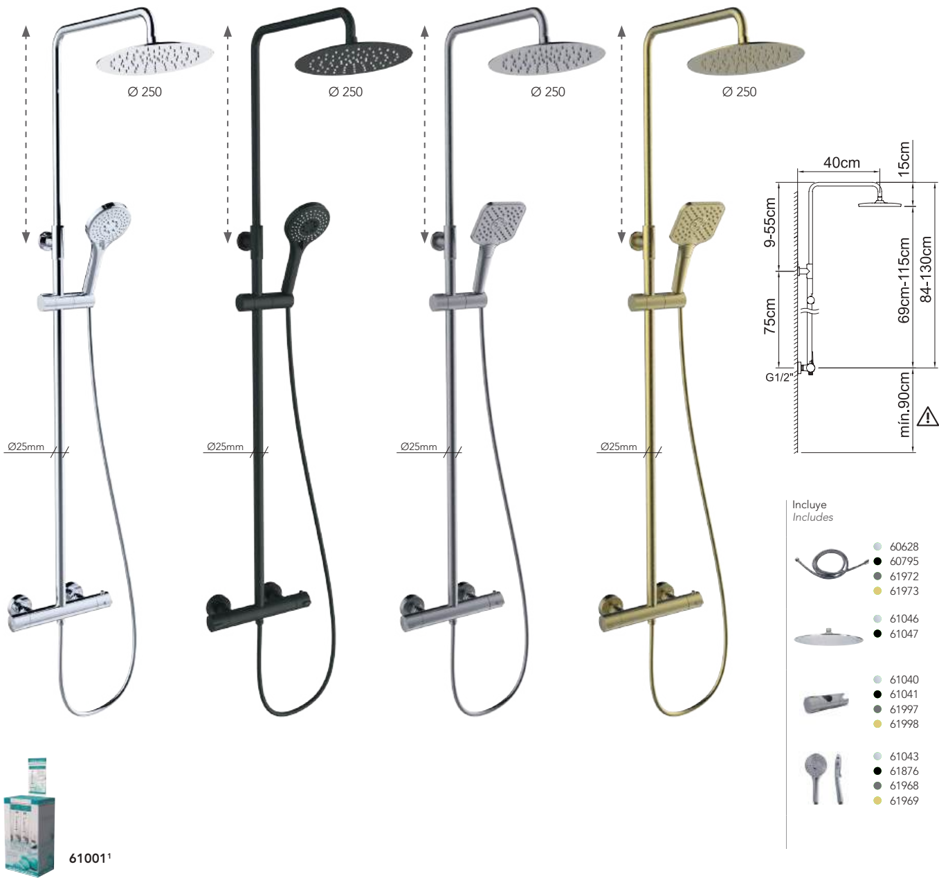
Conjunto de ducha termostática con barra extensible con soporte articulado deslizante. Thermostatic shower set with extendable bar with sliding articulated support.
