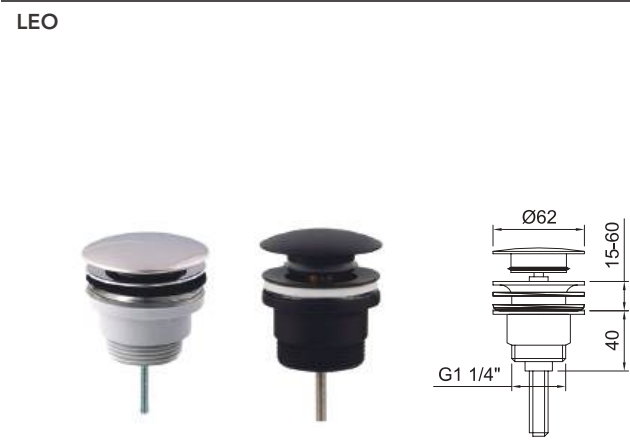
Válvula desagüe universal sistema quick-clac 1 1/4". Pop-up quick-clac 1 1/4".
