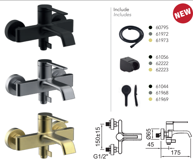
Vasca con doccia monocomando con aeratore e deviatore ceramica. Single-lever bath-shower mixer with aerator and ceramic diverter.
