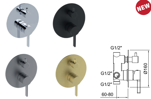
Doccia monocomando da incasso da 1/2". Concealed single-lever shower mixer 1/2".
