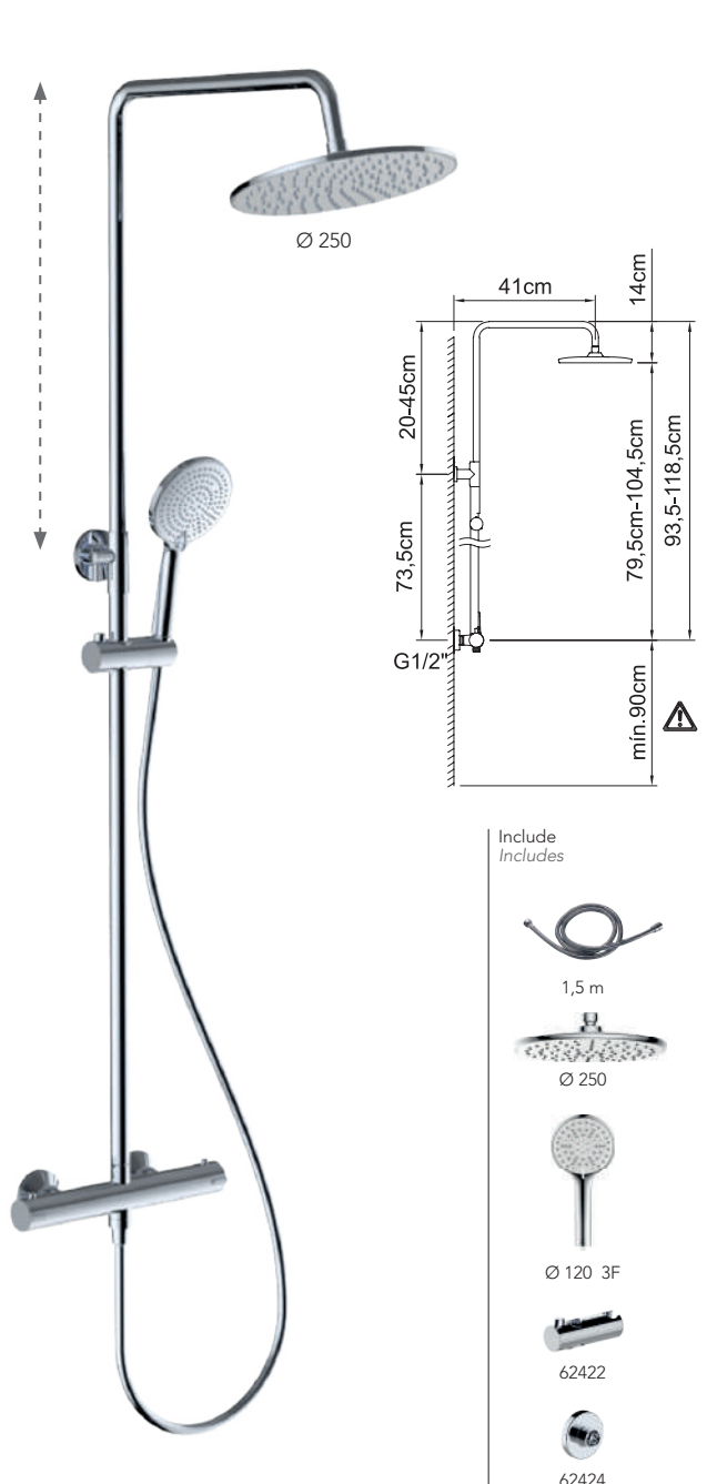
Kit doccia con miscelatore termostatico con asta estraibile con supporto articolato scorrevole. Thermostatic shower set with extendable bar with sliding articulated support.
