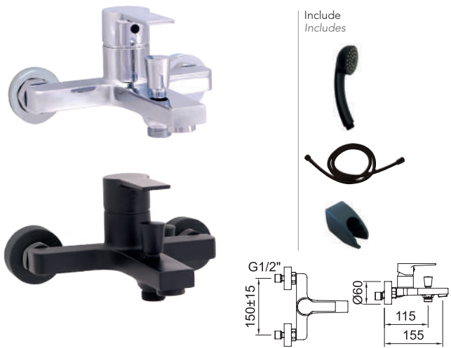
Vasca con doccia monocomando con aeratore e deviatore. Single-lever bath-shower mixer with aerator and diverter.
