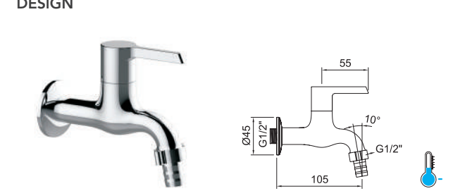
Rubinetto a parete da 1/2" con attacco per tubo di gomma. Wall mounted tap 1/2" with hose fitting.
