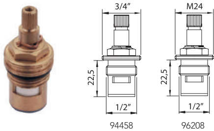
Cartuccia con meccanismo in ceramica. Ceramic headwork.
