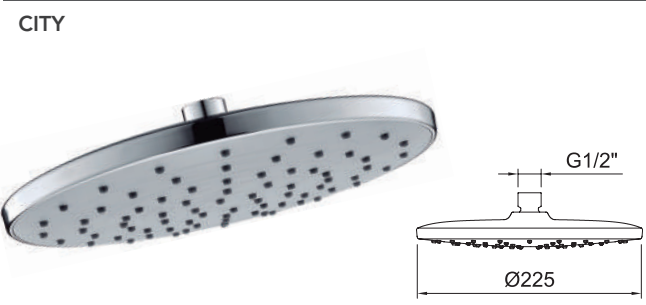
Soffione per doccia City Ø225mm. City head shower Ø225mm.
