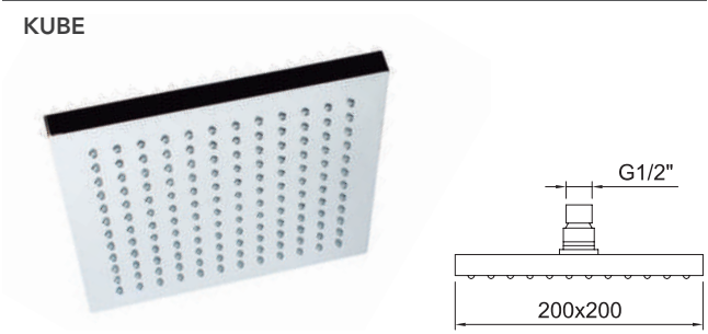
Soffione per doccia Kube 200x200mm. Kube head shower 200x200mm.
