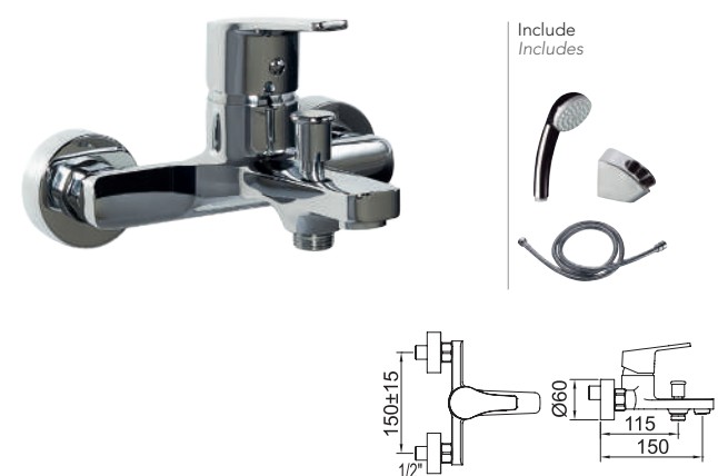
Vasca con doccia monocomando con aeratore e deviatore. Single-lever bath-shower mixer with aerator and diverter.
