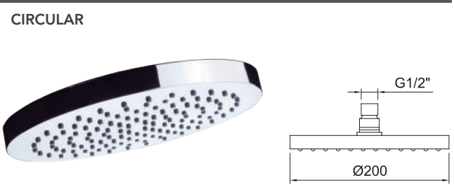
Soffione per doccia Circular Ø200mm. Circular head shower Ø200mm.
