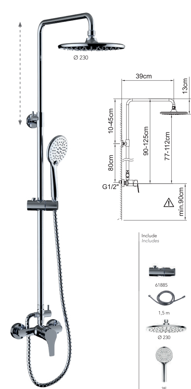
Kit doccia con monocomando con asta estraibile con supporto articolato scorrevole. Single-lever shower set mixer with extendable bar with sliding articulated support.
