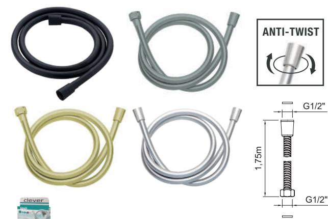
Tubo flessibile per doccia. Hose. 1,75m
