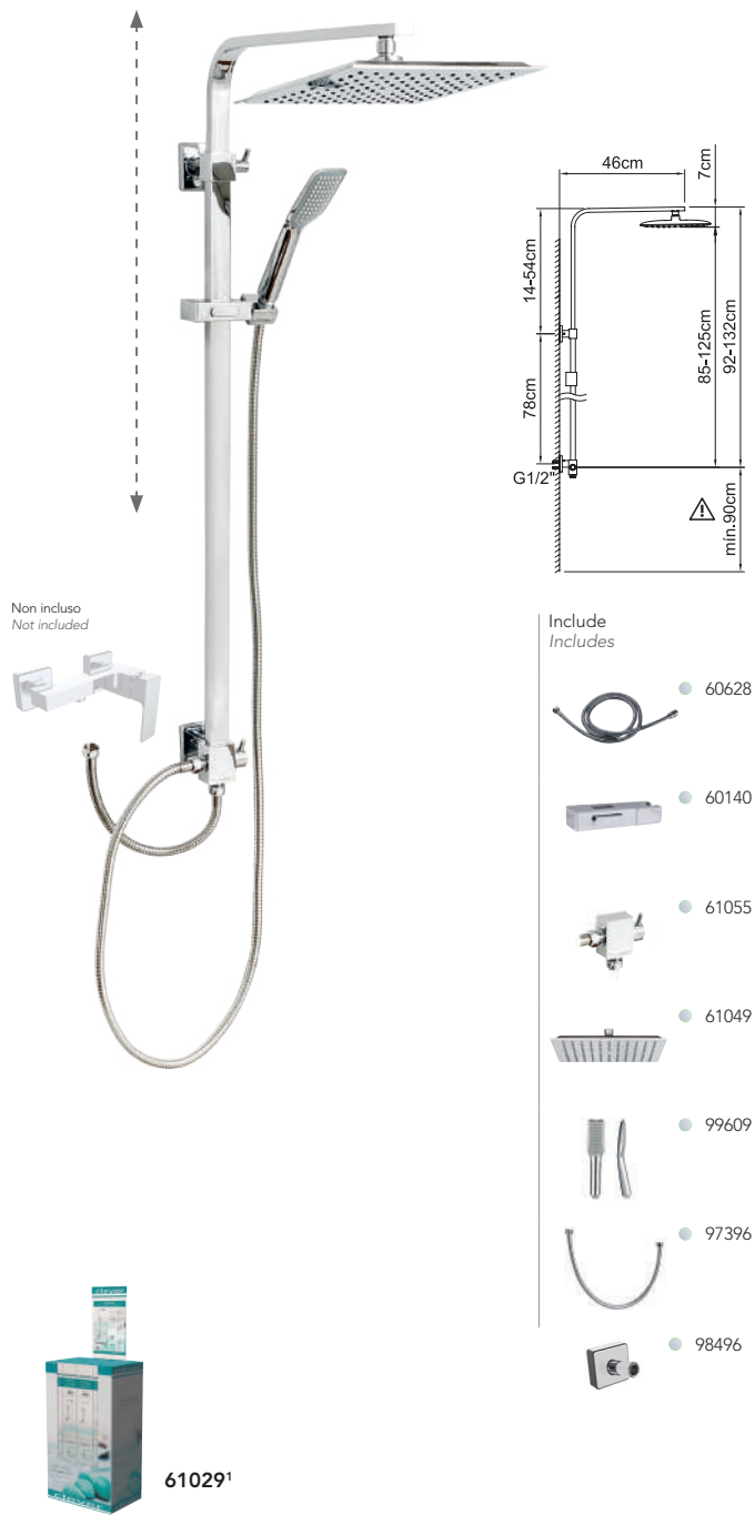
Kit doccia con asta estraibile con supporto articolato scorrevole. Shower set with extendable bar with sliding articulated support.
