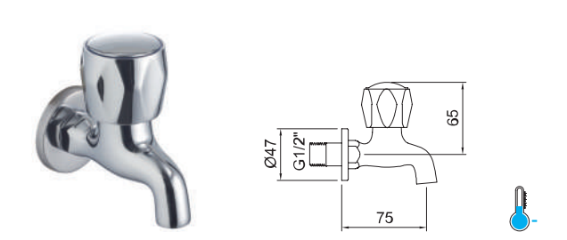
Rubinetto per lavabo a parete da 1/2". Wall mounted basin tap 1/2".
