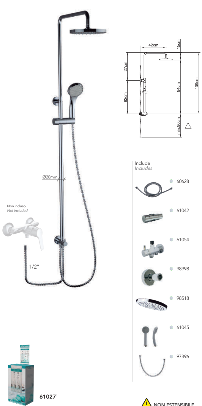
Kit doccia con asta non estraibile con supporto articolato scorrevole. Shower set with non-extendable bar with sliding articulated support.
