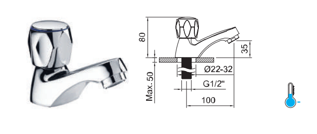
Rubinetto per lavabo da appoggio da 1/2" con aeratore. Deck mounted basin tap 1/2" with aerator.
