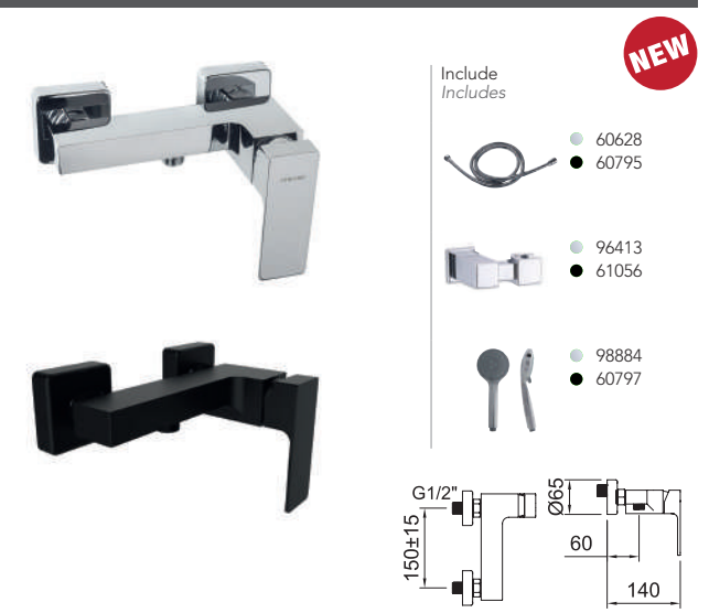
Doccia monocomando. Single-lever shower mixer.
