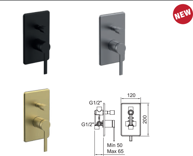
Doccia monocomando da incasso da 1/2". Concealed single-lever shower mixer 1/2".
