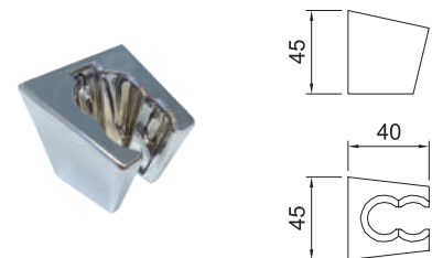
Supporto per doccia di doccia fissa. Fix handset holder.
