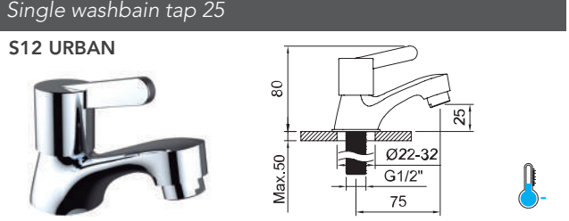
Rubinetto per lavabo da appoggio da 1/2" con aeratore. Deck mounted basin tap 1/2" with aerator.
