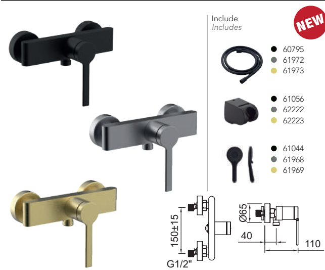
Doccia monocomando. Single-lever shower mixer.
