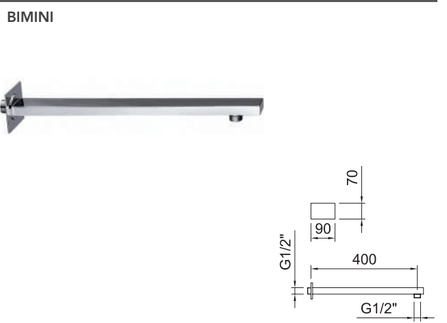
Braccio per soffione a parete Bimini 400 mm. Bimini wall-mounted arm shower 400mm.
