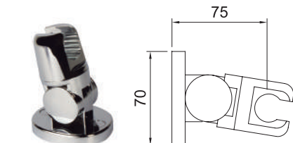
Supporto articolato per doccia. Articulated handset holder.
