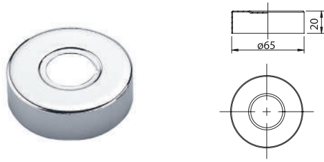
Rosetta con dorso piatto (2 unità). Cromato. Rosette (2 units). Chromed
