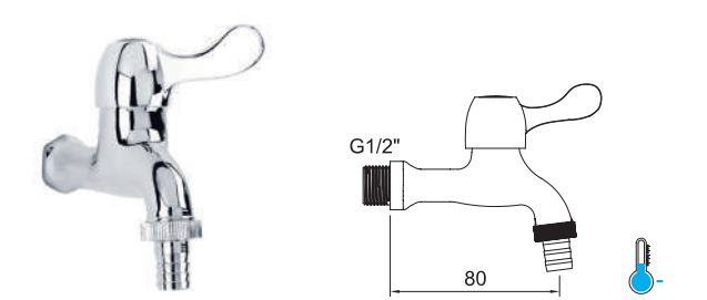
Rubinetto a parete con attacco per tubo di gomma. Wall mounted tap with hose fitting.
