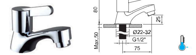
Rubinetto per lavabo da appoggio da 1/2" con aeratore. Deck mounted basin tap 1/2" with aerator.
