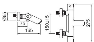
Vasca con doccia termostatica con aeratore e deviatore incorporati nella leva di portata. Thermostatic bath-shower mixer with aerator and and integrated shower diverter.
