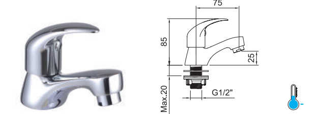
Rubinetto per lavabo da appoggio da 1/2" con aeratore. Deck mounted basin tap 1/2" with aerator.
