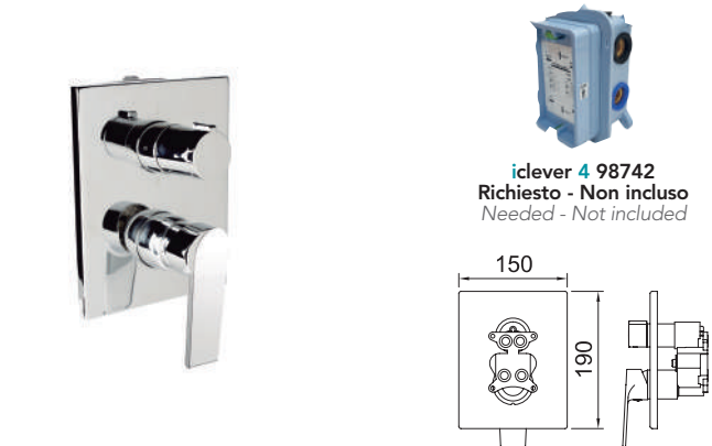
Doccia monocomando da incasso da 1/2". Concealed single-lever shower mixer 1/2".
