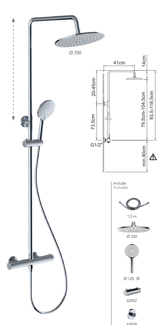
Kit doccia con miscelatore termostatico con asta estraibile con supporto articolato scorrevole. Thermostatic shower set with extendable bar with sliding articulated support.
