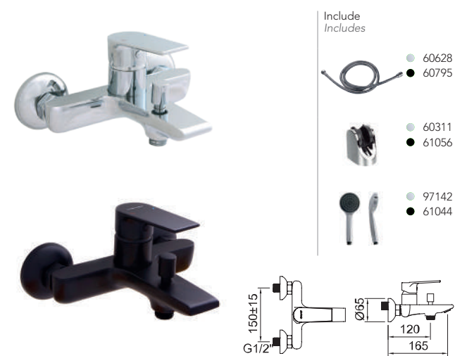
Vasca con doccia monocomando con aeratore e deviatore automatico. Single-lever bath-shower mixer with aerator and automatic diverter.
