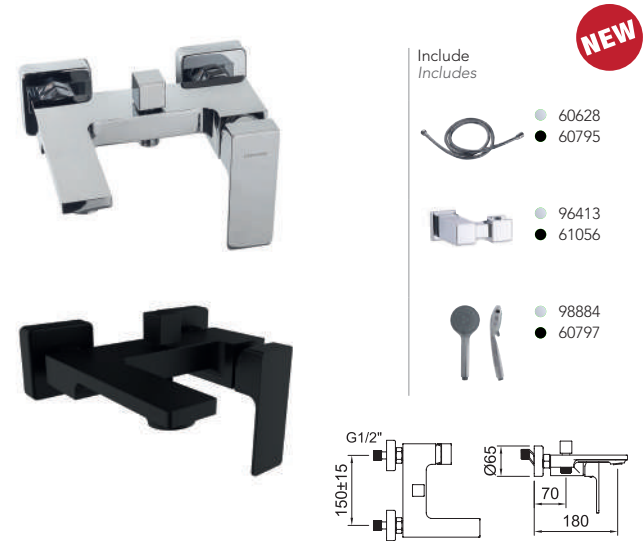
Vasca con doccia monocomando con aeratore e deviatore automatico. Single-lever bath-shower mixer with aerator and automatic diverter.
