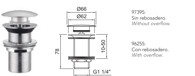
Válvula desagüe sistema quick-clac 1 1/4". Pop-up quick-clac 1 1/4".
