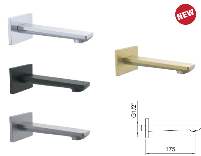
Caño baño mural. Bath spout.
