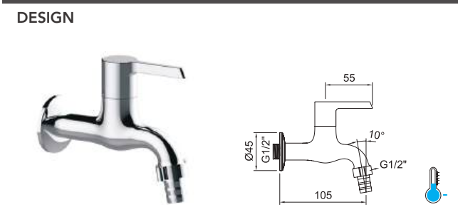
Grifo mural 1/2\" con accesorio manguera.
