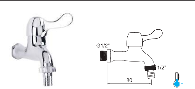
Grifo mural con accesorio manguera.
