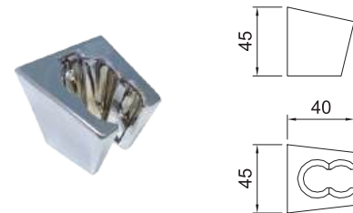
Soporte teléfono de ducha fijo. Fix handset holder.
