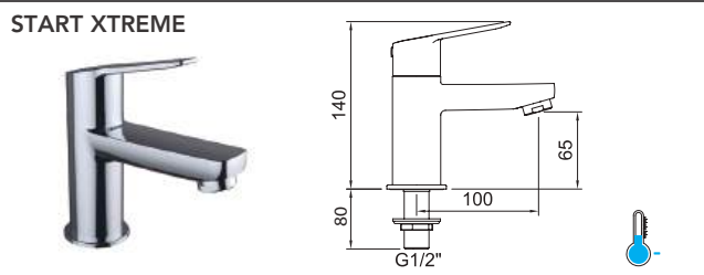
Grifo lavabo repisa 1/2\" con aireador.
