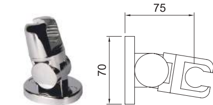
Soporte teléfono de ducha articulado. Articulated handset holder.
