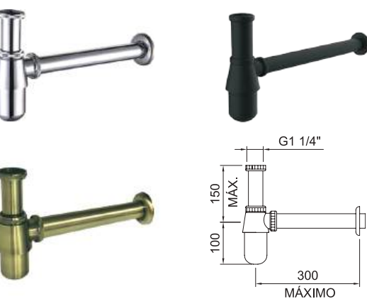
Sifón de botella 1 1/4" con tubo de Ø32mm. Bottle trap 1 1/4" with tube Ø32mm.
