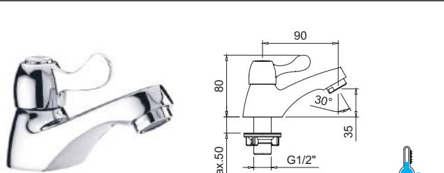
Grifo lavabo 1/2\"repisa con aireador.
