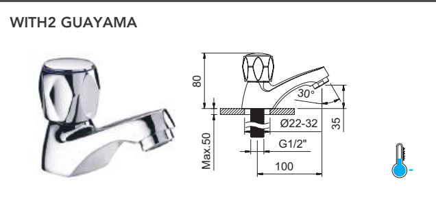
Grifo lavabo repisa 1/2\" con aireador.
