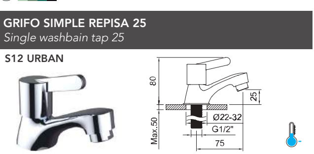
Grifo lavabo repisa 1/2\" con aireador.
