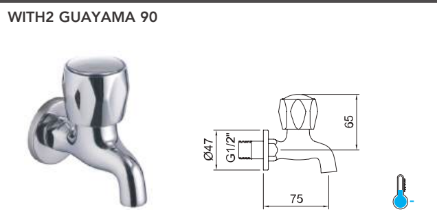
Grifo lavabo mural 1/2\".
