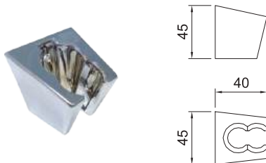
Supporto per doccia di Doccetta fissa. Fix handset holder.
