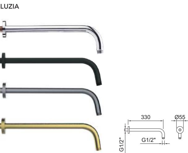
Braccio per soffione a parete Luzia da 330 mm. Luzia wall-mounted arm shower 330mm.
