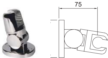
Supporto articolato per doccia. Articulated handset holder.
