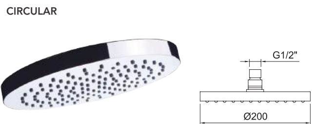
Soffione per Doccetta Circular Ø200mm. Circular head shower Ø200mm.
