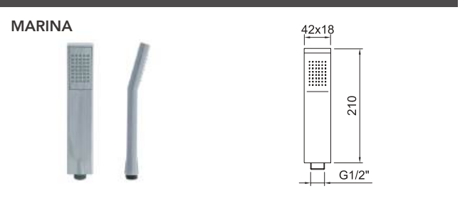
Doccetta Marina. Marina shower handset.
