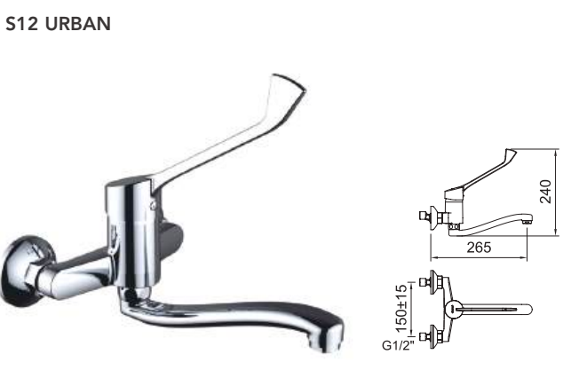
MISCELATORE DA CUCINA A PARETE CON RUBINETTO INFERIORE CON LEVA CLINICA Wall mounted sink mixer with medical lever
