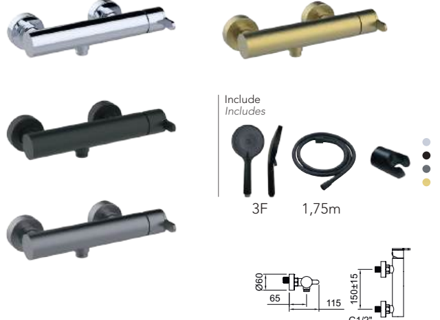
Doccia monocomando. Single-lever shower mixer.
