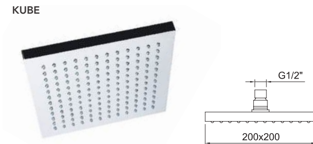
Soffione per Doccetta Kube 200x200mm. Kube head shower 200x200mm.
