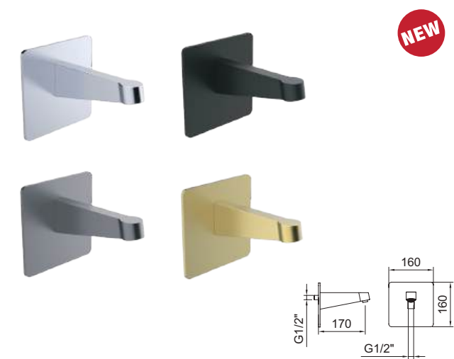
Braccio per soffione a parete. Wall-mounted arm shower.
