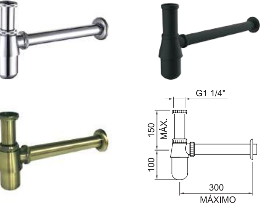
Sifone a bottiglia da 1 1/4" con tubo da Ø32mm. Bottle trap 1 1/4" with tube Ø32mm.
