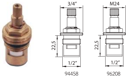
Cartuccia ceramica. Ceramic headwork.
