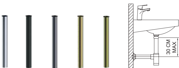
Prolunga per sifone. Bottle trap extension.
