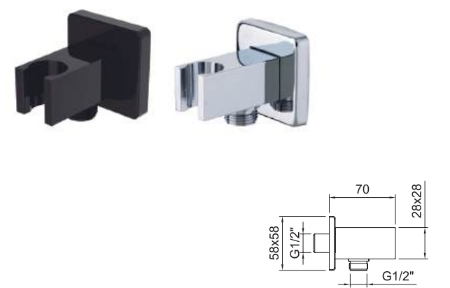
Uscita per tubo flessibile da parete con supporto. Wall hose outlet with holder.
