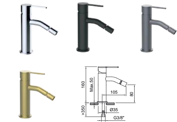
Bidet monocomando con aeratore a snodo e tubi flessibili da 3/8" >350mm. Single-lever bidet mixer with swivel aerator and flexible hoses 3/8" >350mm.
