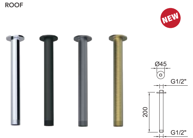
Braccio per soffione a soffitto da 200 mm. Roof ceiling arm shower 200mm.
