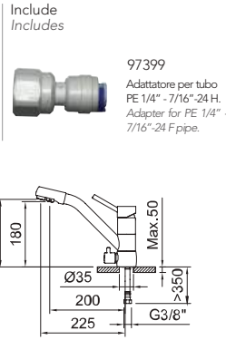
MISCELATORE DA CUCINA A 3 VIE PER IMPIANTI DI TRATTAMENTO DELL'ACQUA 3 way sink mixer for water quality equipment
