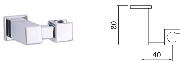
Supporto articolato per doccia. Articulated handset holder.
