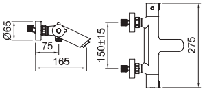
Vasca con doccia termostatica con aeratore e deviatore incorporati nella leva di portata. Thermostatic bath-shower mixer with aerator and and integrated shower diverter.
