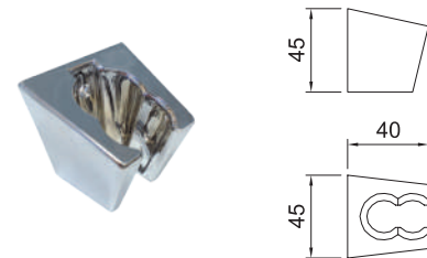
Suporte fixo para chuveiro de mão. Fix handset holder.
