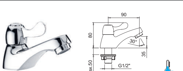
Torneira de banca para lavatório 1/2" com areador. Deck mounted basin tap 1/2" with aerator.
