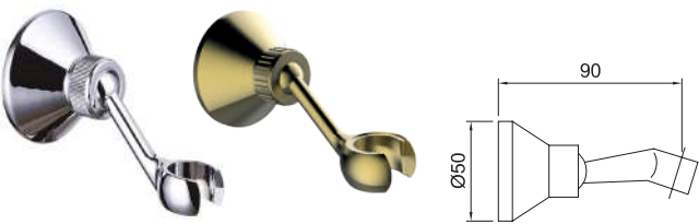
Suporte articulado para chuveiro de mão. Articulated handset holder.
