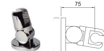
Suporte articulado para chuveiro de mão. Articulated handset holder.
