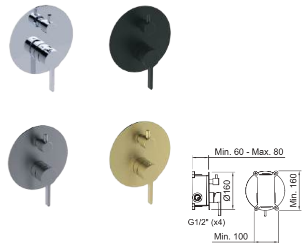
Duche monocomando de embutir 1/2". Concealed single-lever shower mixer 1/2".
