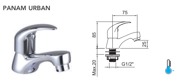
Torneira de banca para lavatório 1/2" com areador. Deck mounted basin tap 1/2" with aerator.
