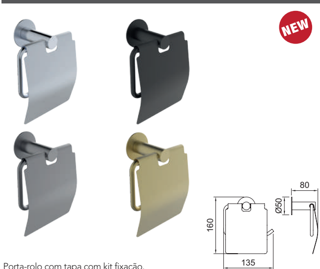
Porta-rolo com tampa com kit fixação. Toilet roll with cover with fixing kit.
