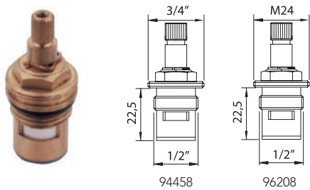
Cartucho cerâmico. Ceramic headwork.
