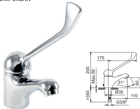
LAVATÓRIO COM MANETE GERONTOLÓGICA Basin mixer with medical lever
