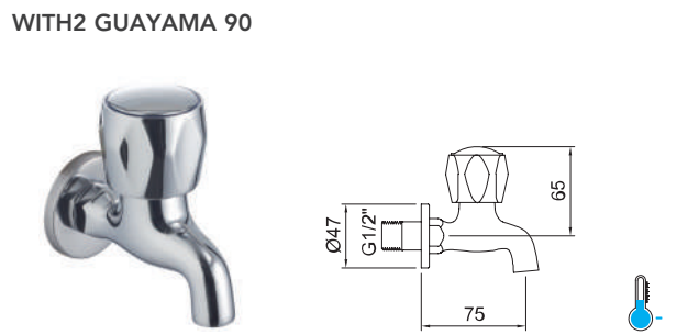
Torneira mural para lavatório 1/2". Wall mounted basin tap 1/2".
