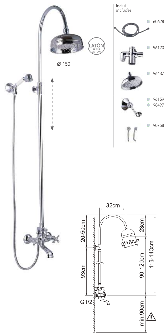
Conjunto de banheira-duche bicomando com barra extensível e suporte articulado. Two-handed bath-shower set with extendable bar and articulated support.
