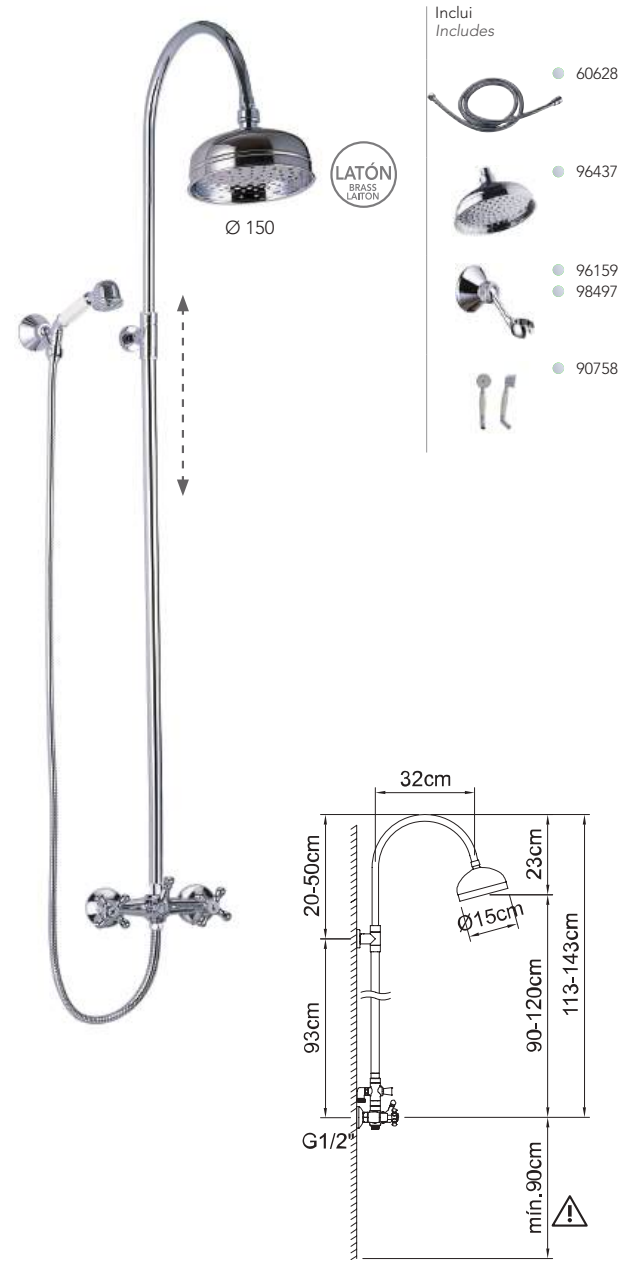
Conjunto de duche bicomando com barra extensível e suporte articulado. Two-handed shower set with extendable bar and articulated support.
