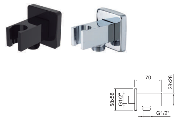
Saída para flexível mural com suporte. Wall hose outlet with holder.
