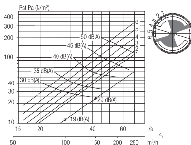
Graphique et plaque de réglage WK 600-1
