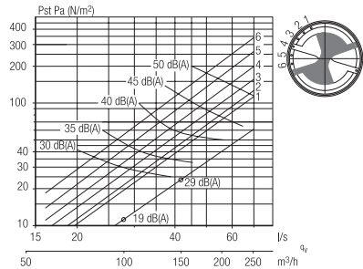
Einstellgraphiken -platte WK 600-1
