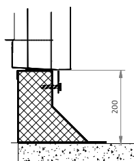
Bevestiging aan buitenzijde dakkap. (aluminium dakopstand; afgebeeld BDOEAR)
