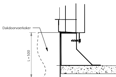
Aluminium dakdoorvoerkoker BDOKAD (optioneel)
