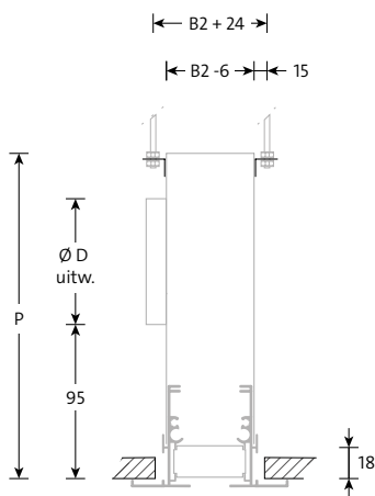
rechte plenumbox sparingmaat = B2
