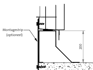
Bevestiging aan binnenzijde dakkap. (aluminium dakopstand; afgebeeld BDONAD)
