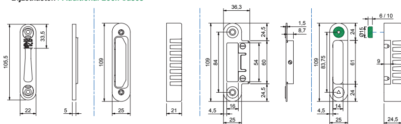
Verstelbare Sluitplaat Haakschoot Art. 600357 Adjustable Strike for Hookbolt
