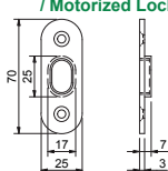
Magneet voor MPS (Auto)Motortronic Art. 200076 Magnet for MPL's (Auto)Motortronic
